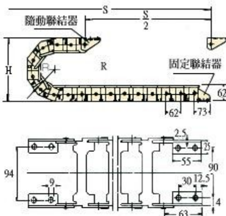
TLP40拖鏈 開扣型
