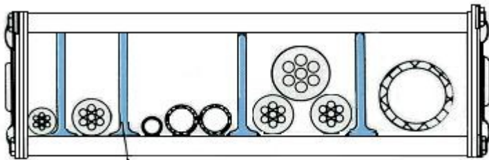
塑料-隔條
