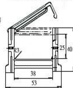
TLP30拖鏈 開扣型
