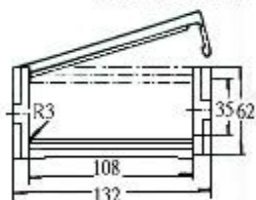
TLP40拖鏈 開扣型
